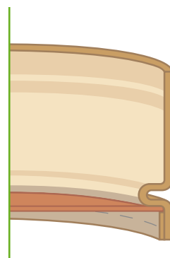
MDF-Boden formschlüssig zwischen Sicke und Stoß-Pappring geklemmt und geheftet
